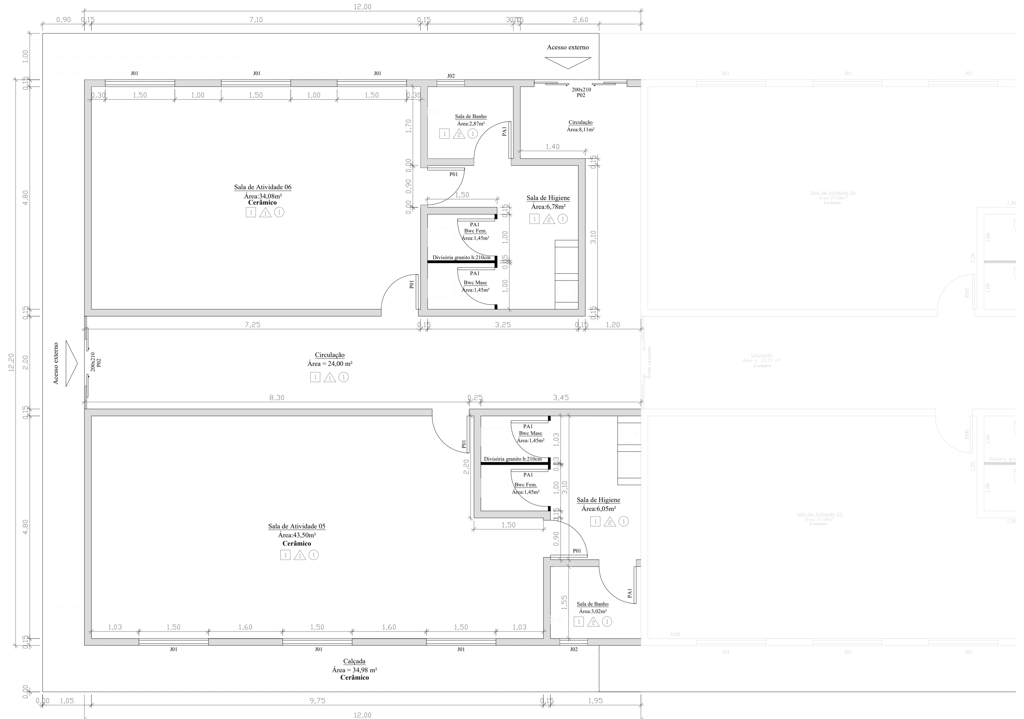
PLANTA BAIXA Esc: 1/50
