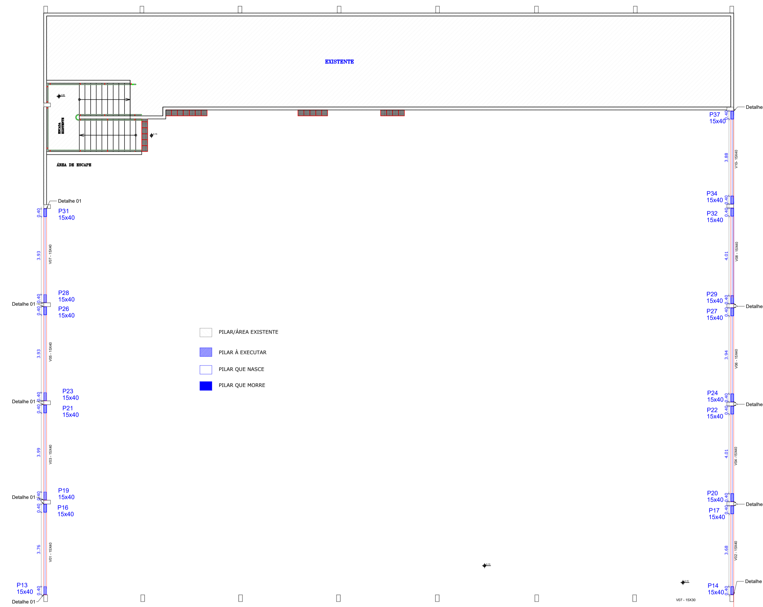
PLANTA BAIXA ESTRUTURAL - NÍVEL 7,04m CINTAMENTO
