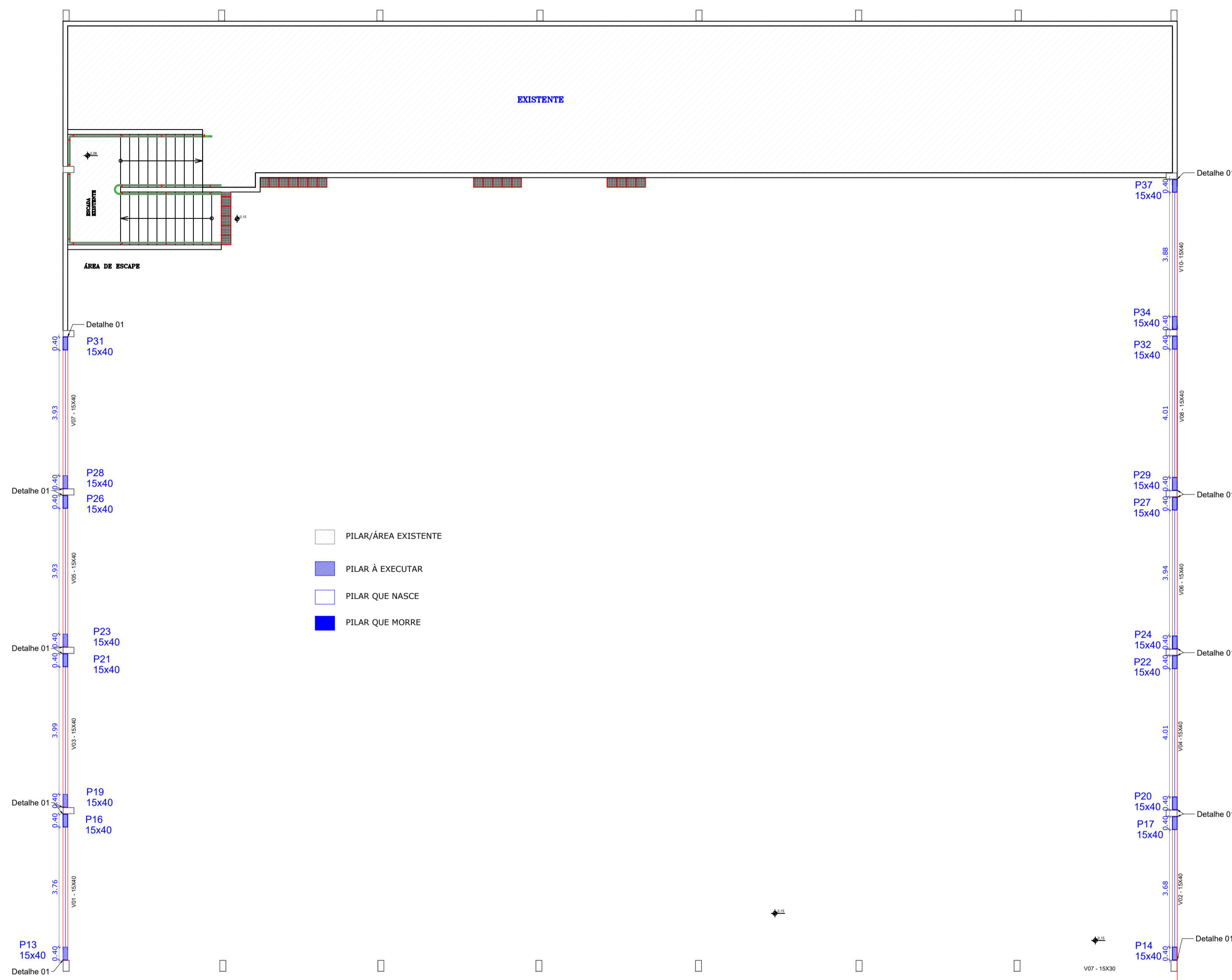
PLANTA BAIXA ESTRUTURAL - NÍVEL 3,69m INTERMEDIÁRIO
