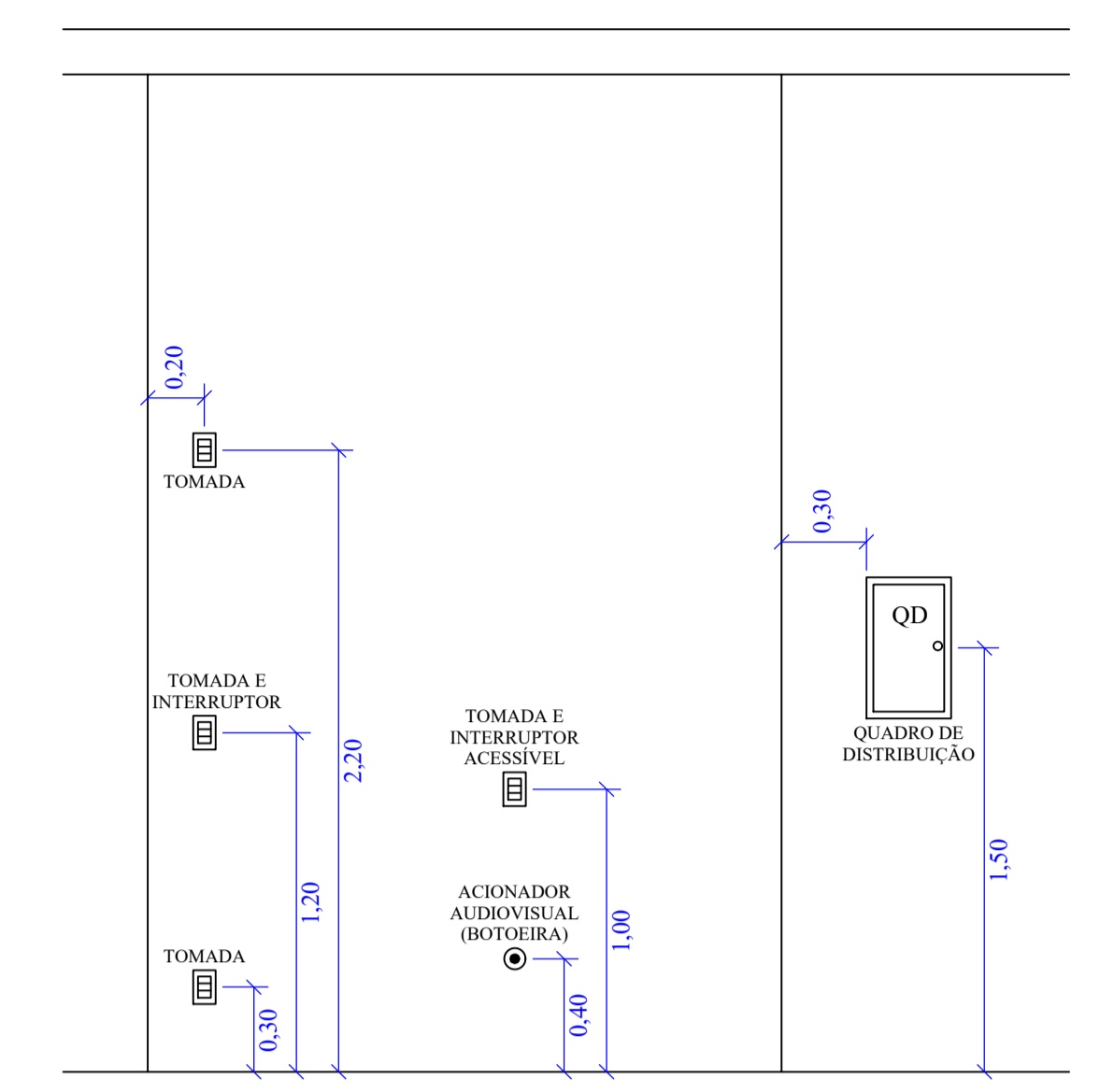
Detalhe Típico de Posicionamento Escala 1:25
