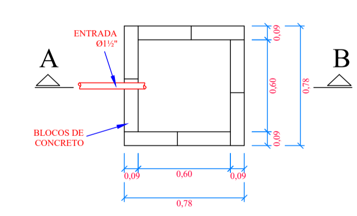
PLANTA BAIXA
