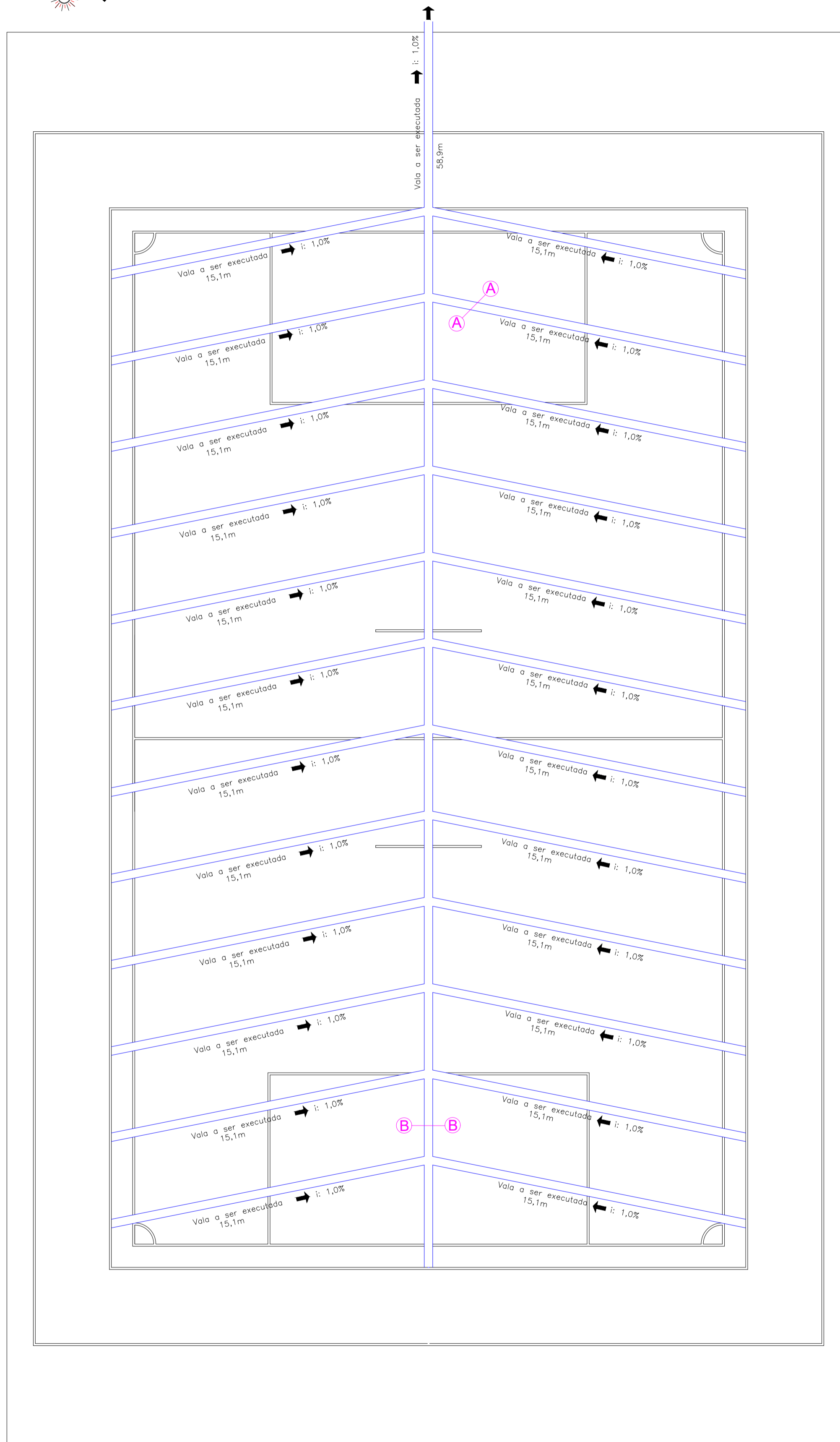
PLANTA BAIXA DRENAGEM - VALAS Escala: 1/150
