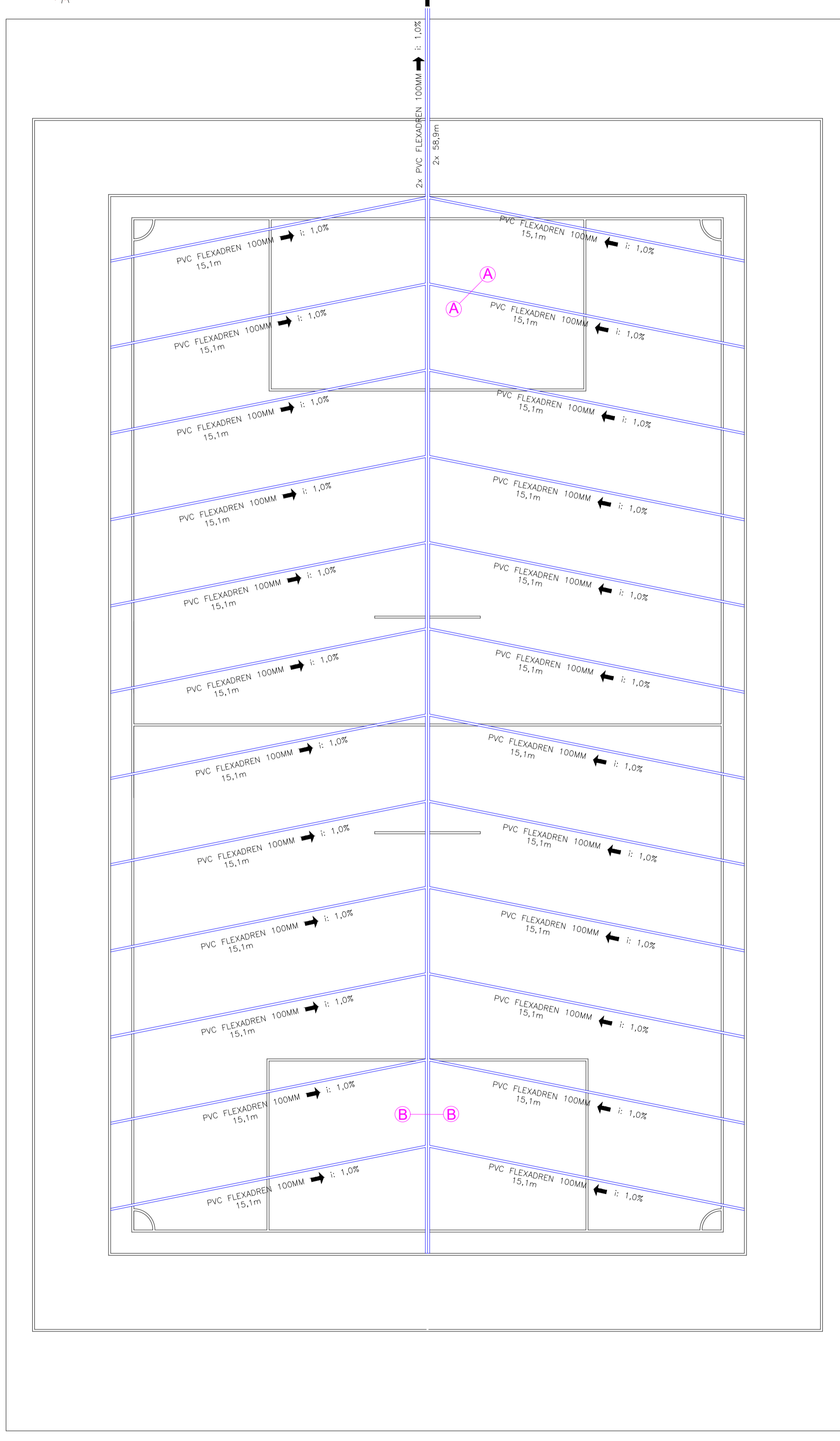
PLANTA BAIXA DRENAGEM - TUBULAÇÃO Escala: 1/150
