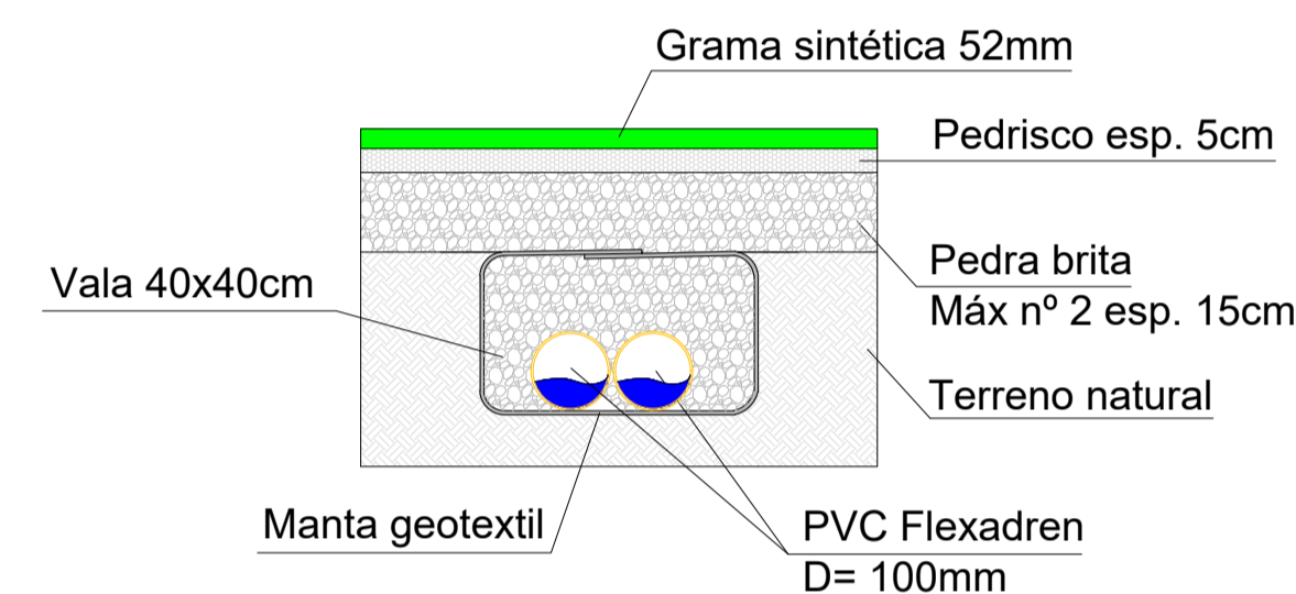
CORTE B-B ESC. 1:20
