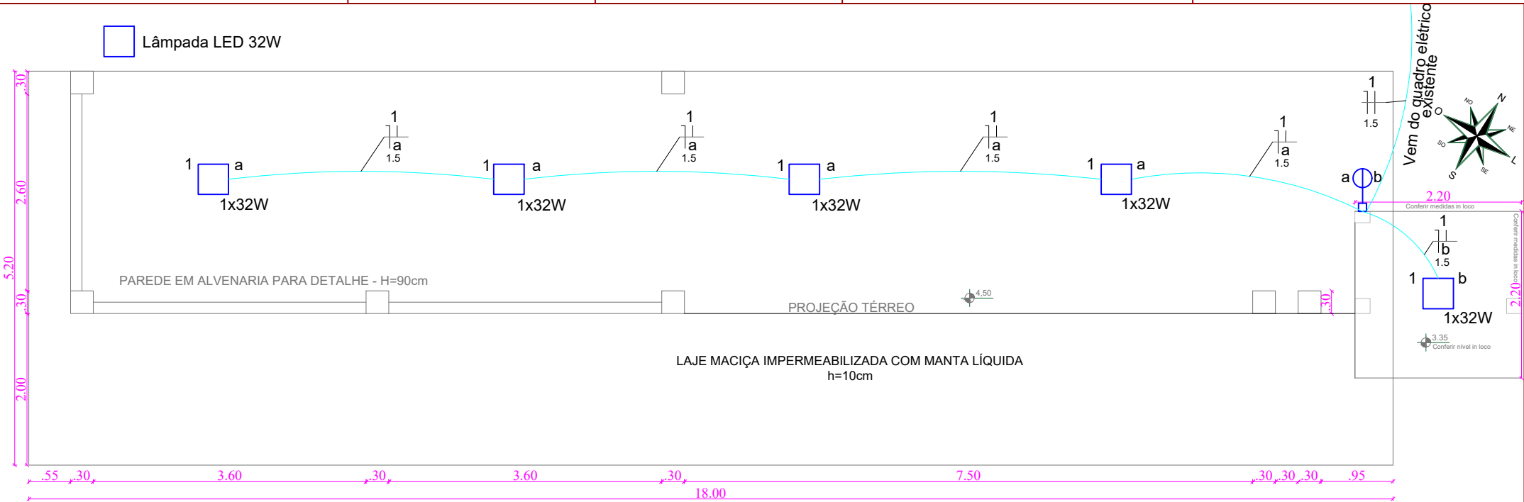
PLANTA BAIXA - ELÉTRICO ESC.: 1/50
