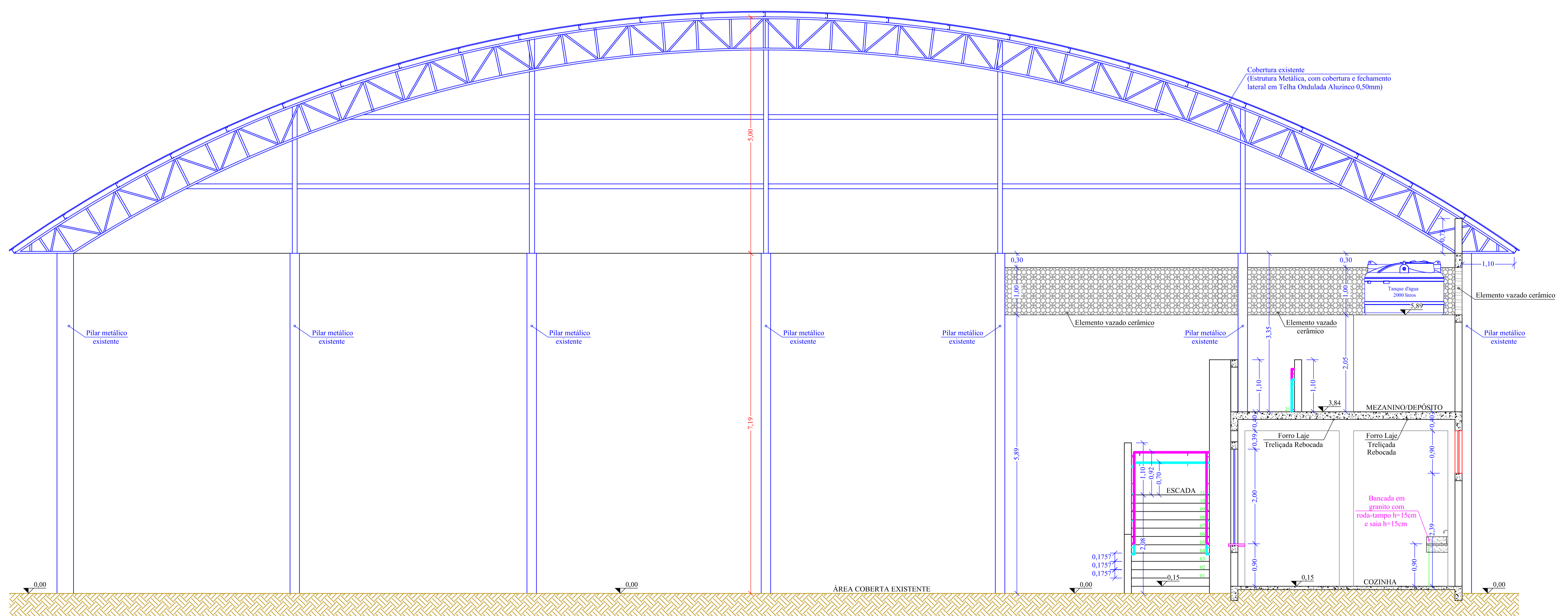
Corte DD Escala 1:50
