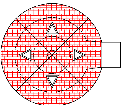
PROJETO ARQUITETÔNICO - PLANTA DE COBERTURA QUIOSQUE C/ CHURRASQUEIRA AREA = 8,04 m 2
