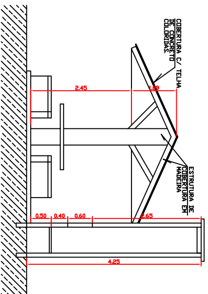
CORTE A-A
