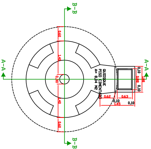
PROJETO ARQUITETÔNICO - PLANTA BAIXA QUIOSQUE C/ CHURRASQUEIRA AREA = 8,04 m 2
