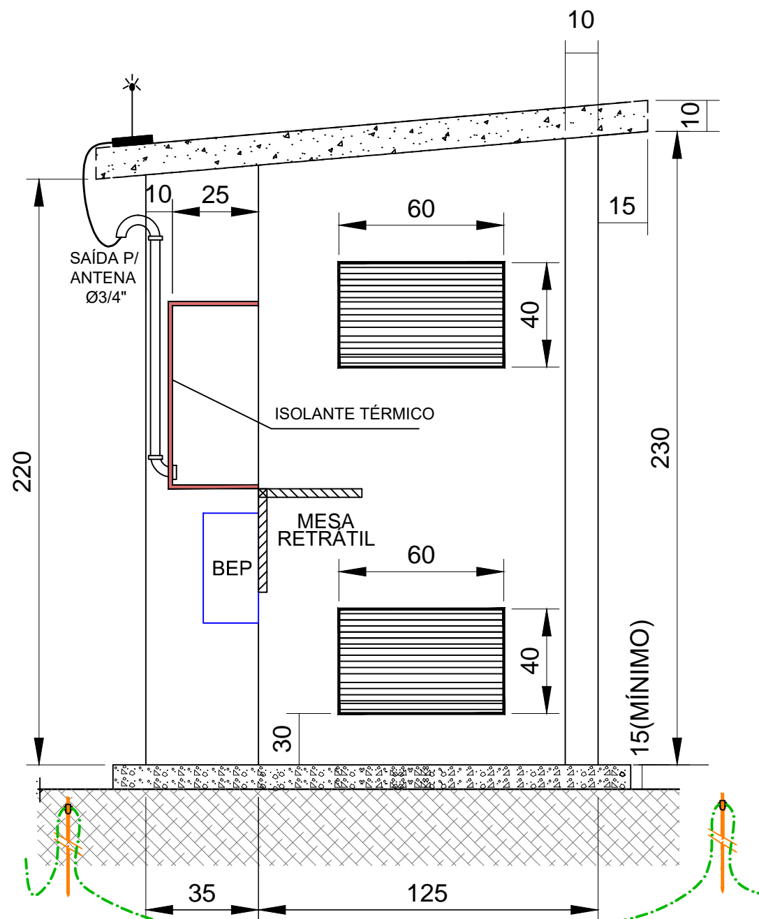
CORTE B-B'
