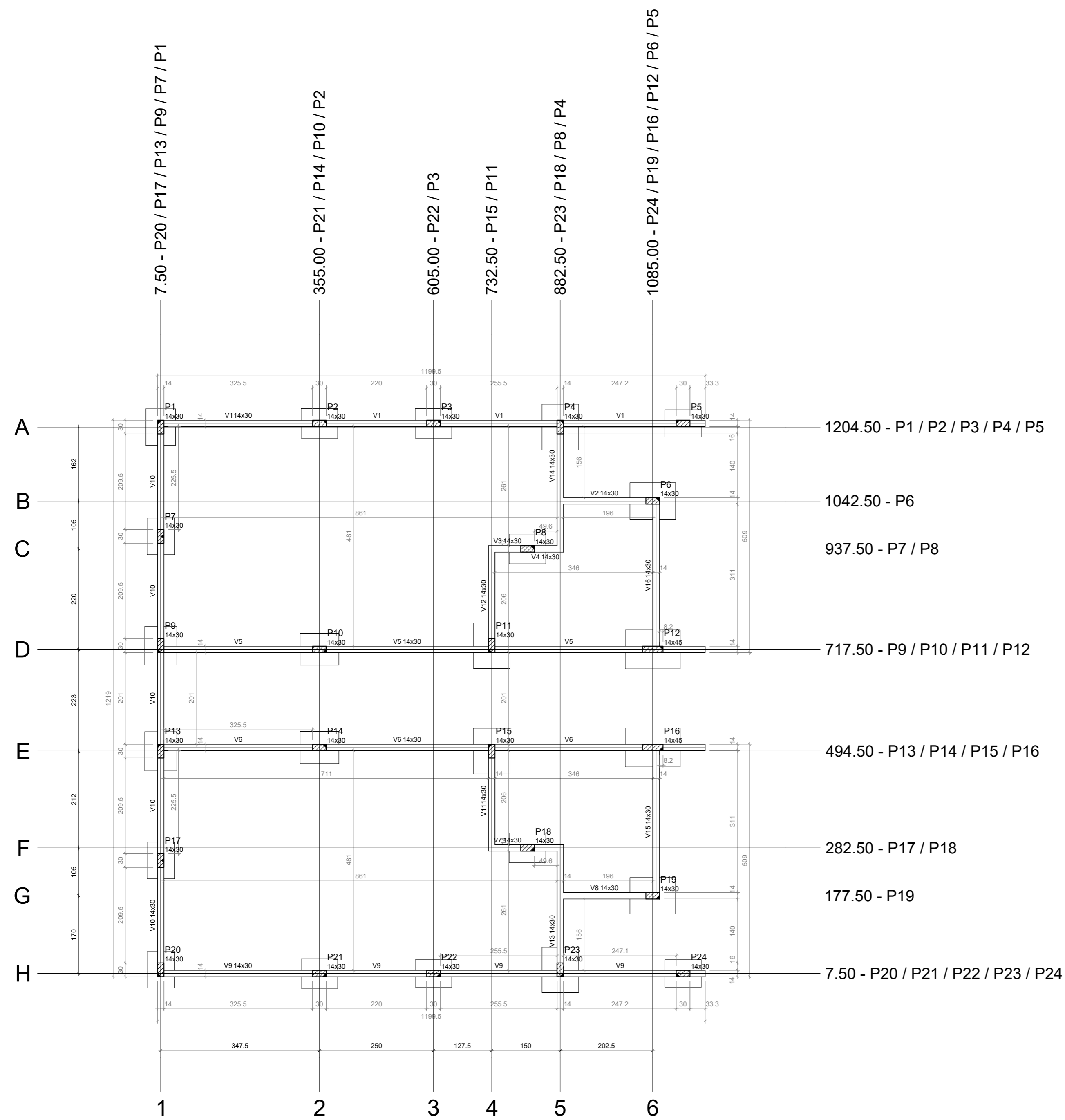
Forma do Vigas Baldrame (Nível 0) escala 1:50
