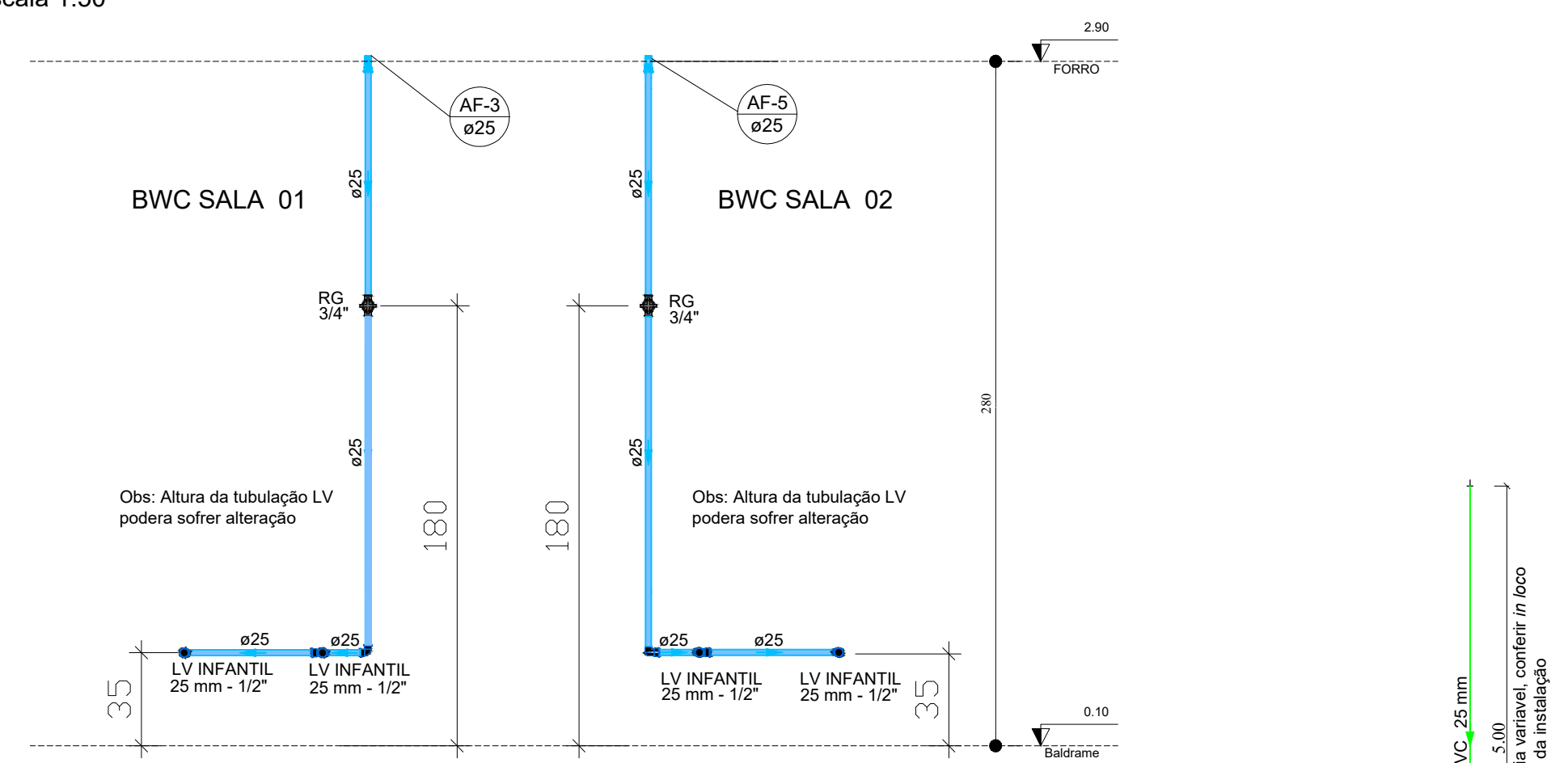
VISTA LAVATÓRIOS Escala 1:50
