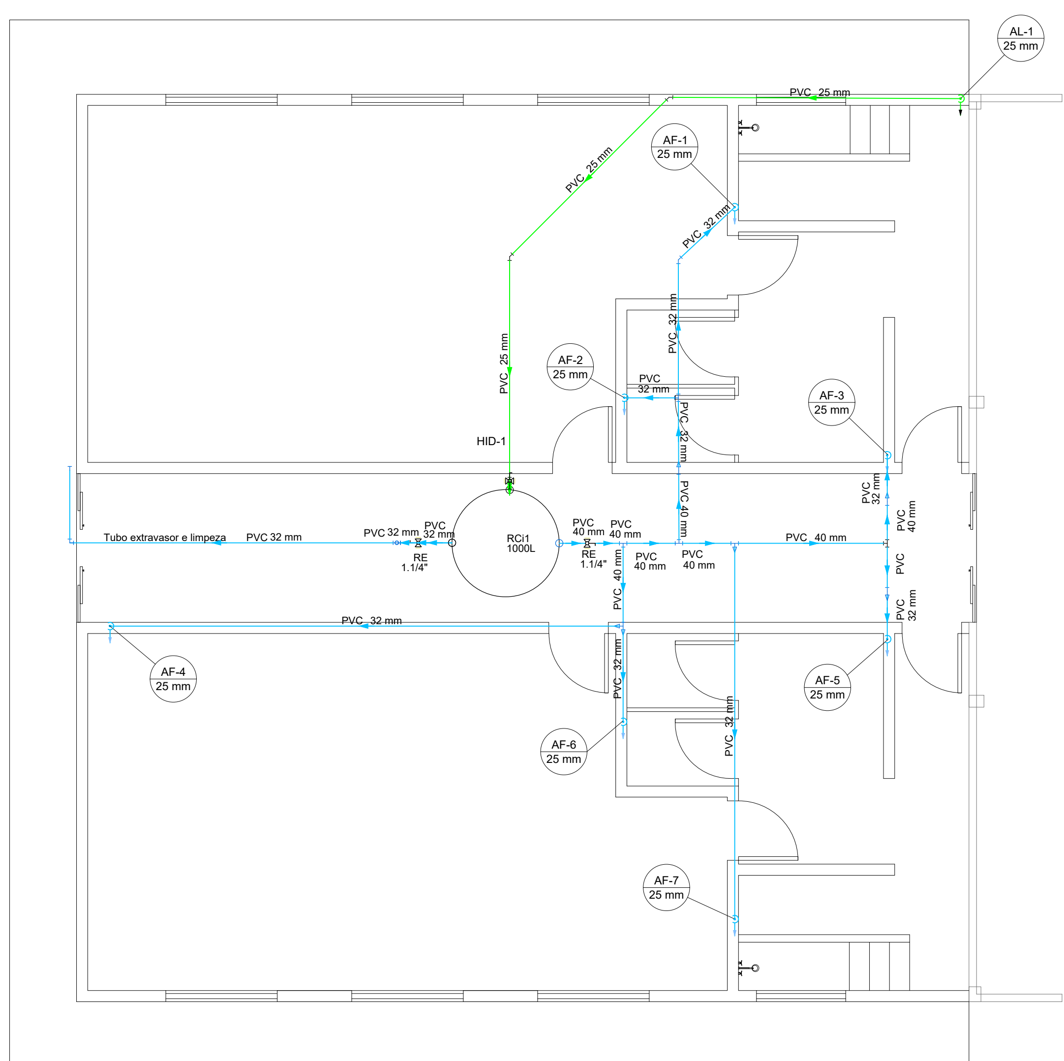
PLANTA BAIXA HIDRÁULICA BARRILETE Esc.: 1:50
