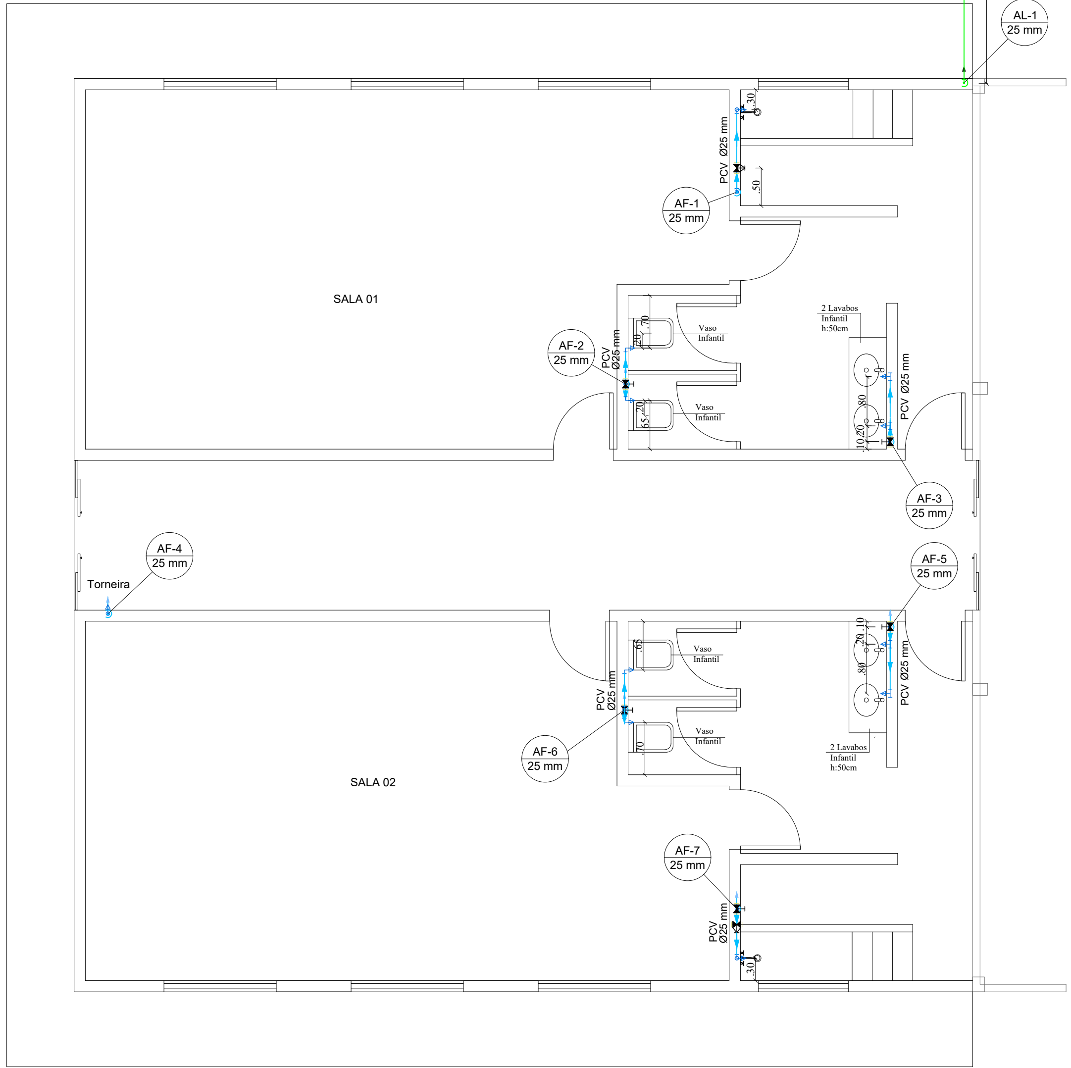
PLANTA BAIXA HIDRÁULICA TÉRREO Esc.: 1:50
